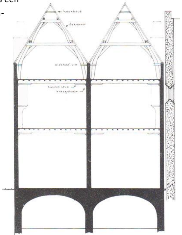
Afb. 9 Reconstructie van de dwarsdoorsnede van de huizen rond 1500.
