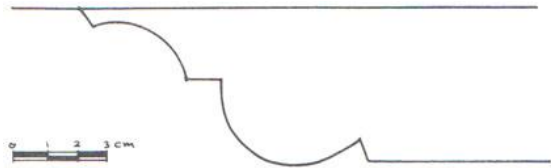
Afb. 10. Profiel van de sleutelstukken van de moerbalken Afb. 11 Profiel van de kraagstenen onder de moerbalken
