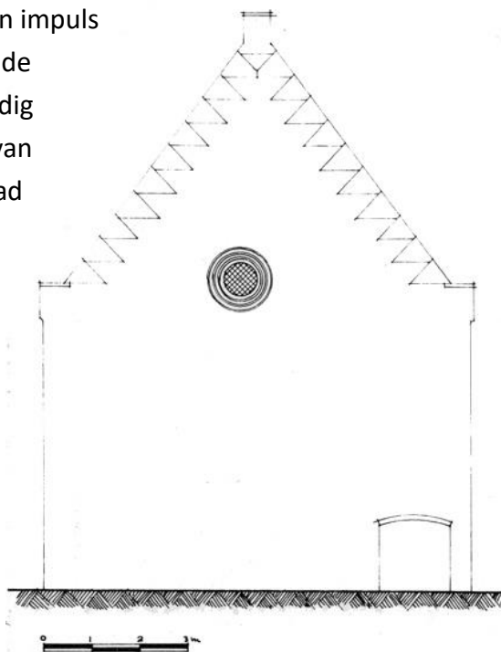
Afb. 25 Reconstructie van de oostgevel van de Lievevrouwekapel
