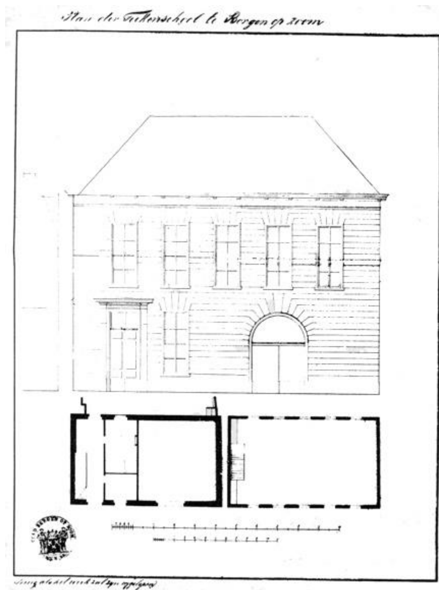
Afb 28 Plan tekening voor de verbouwing van de Korenwaag in 1852.
