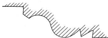
19. Profiel van een balksleutel In het huis Korte :Meestraat 16 (Tekening J. W.).
