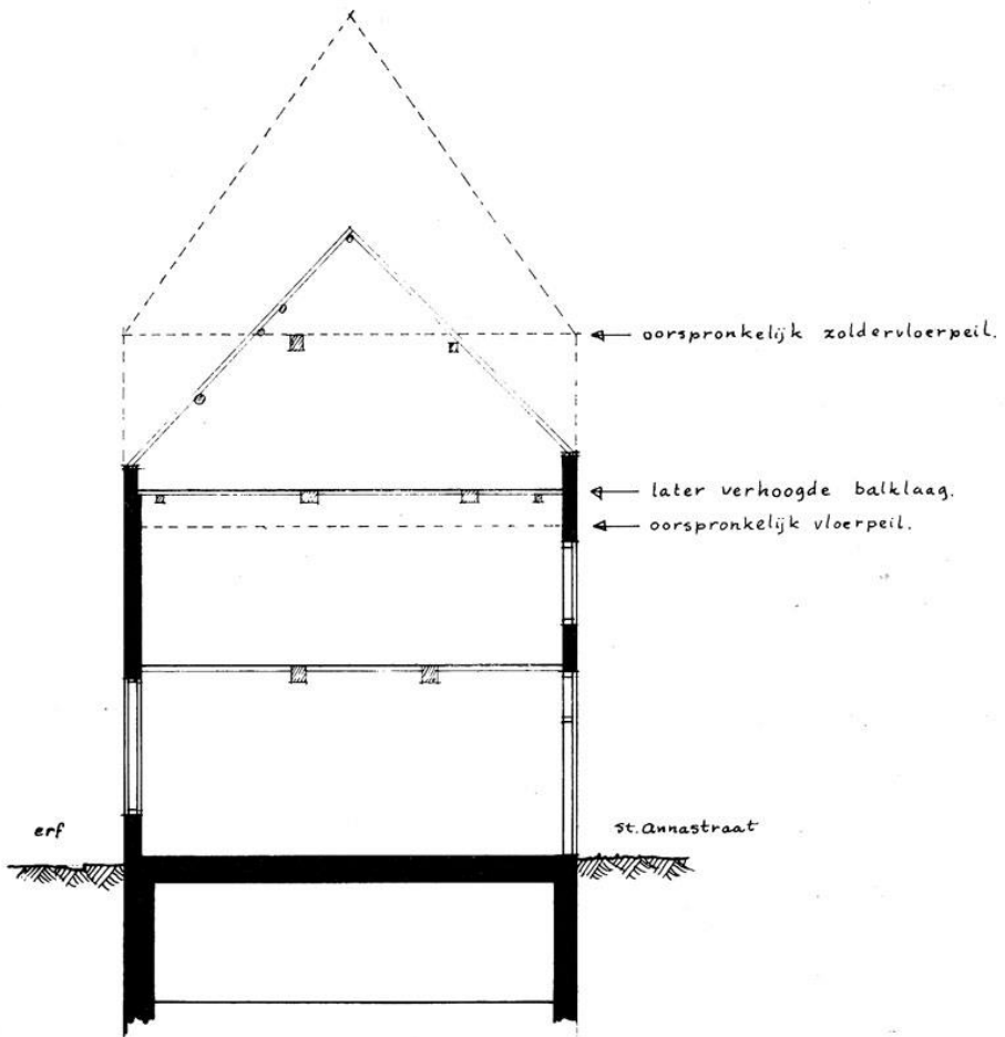
23. Dwarsdoorsnede over het pand Sint Annastraat 20 (Tekening J. W.).
