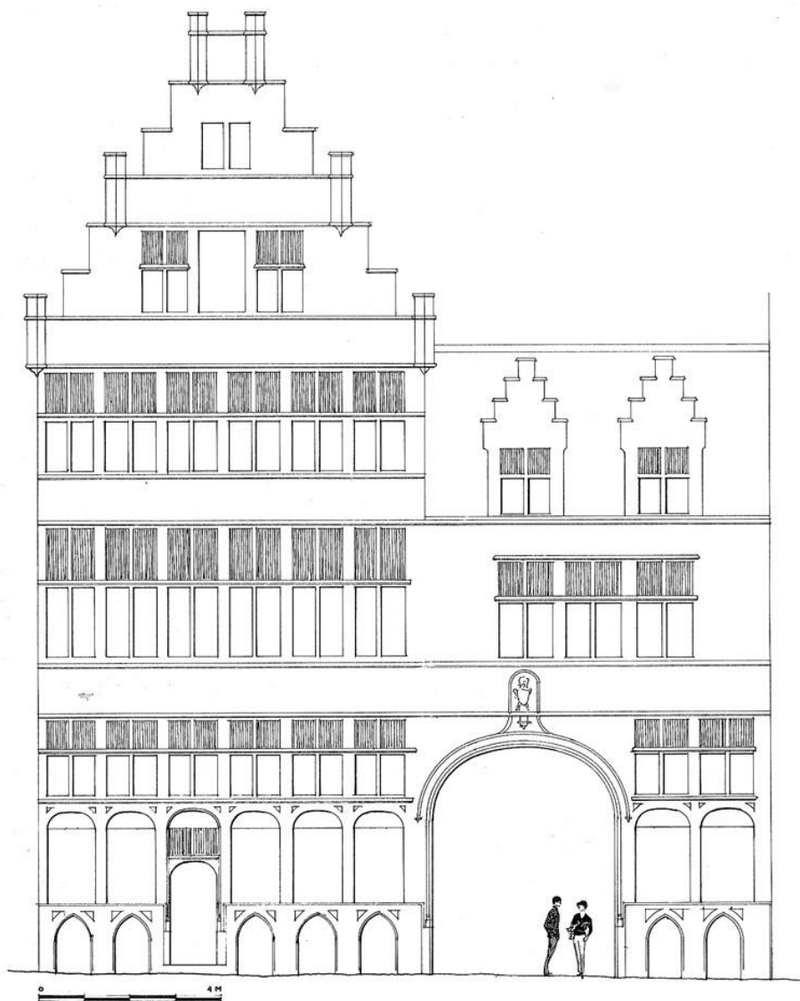
17 Reconstructie van de voorgevels van de huizen Grote Markt 38 en L (Drak en De Olifant) 16e eeuw (Tekening J. W.).
