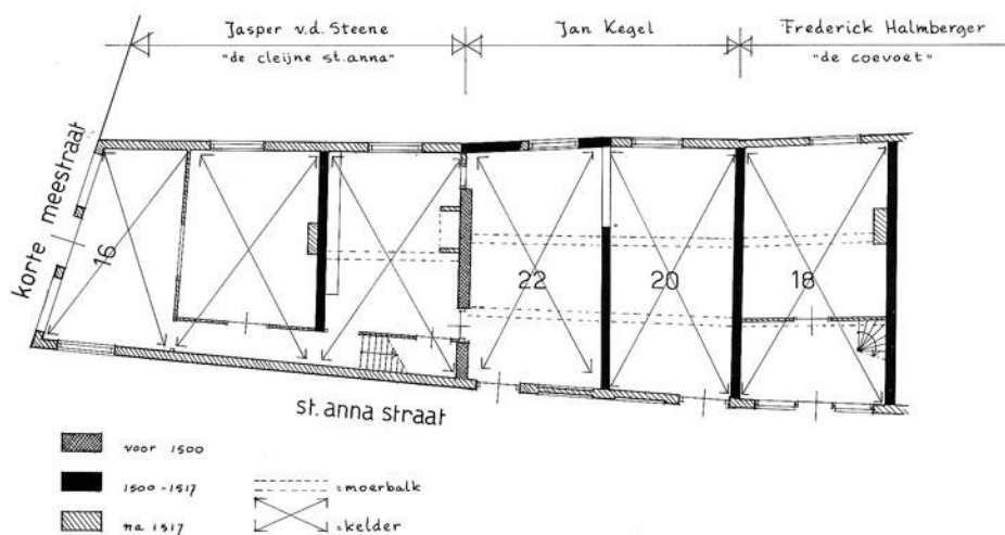
20. Grondplan van de huizen hoek Sint Annastraat-Korte Meestraat (Tekening J. W.).
