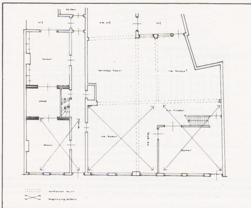
Indeling van de begane grondverdieping in 1946 (tekening ir. J. Weyts)
