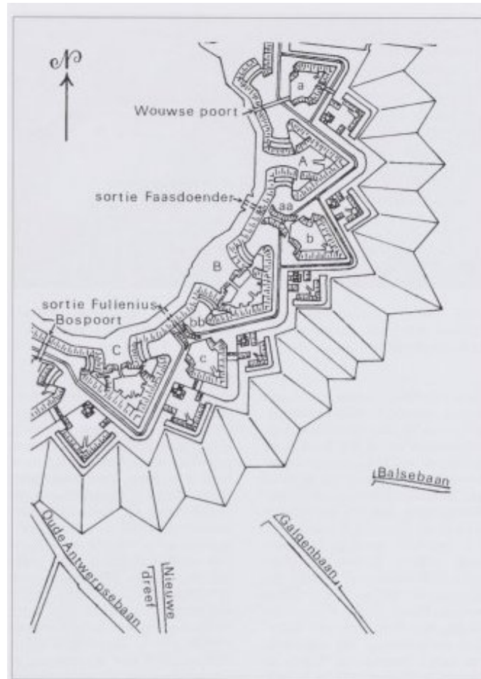
Afh. 11. Het Hoge Front van de vesting. A=bastion William; B=bastion Pucelle, C=bastion Coehoorn; a=ravelijn Wouw, b=ravelijn Wassenaar; c=ravelijn Dedem; aa en bb zijn caponnières (een caponnière is een aarden uitbouw in een vestinggracht). Deze kaart, getekend door Jan Bos, is ontleend aan Merck toch hoe sterck, geschreven door W.A. van Ham, Bergen op Zoom 1982, p. 123.
