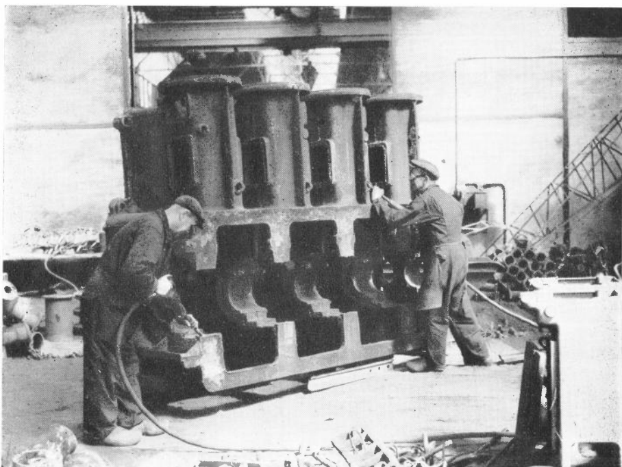
HET AFBRAMEN VAN EEN MACHINEFRAME - GEWICHT CA. 6 TON
