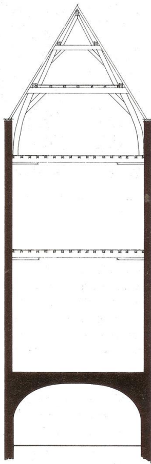
32. Lievevrouwestraat 24. Dwarsdoorsnede.
