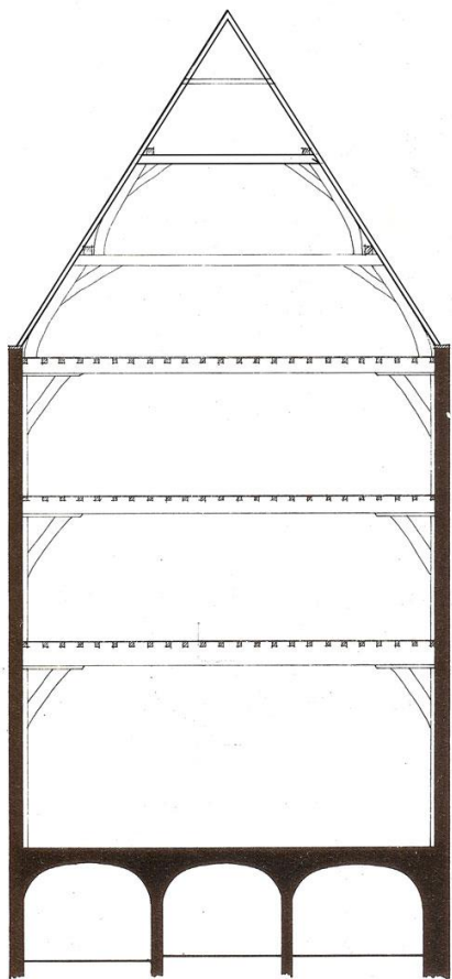
31. Grote Markt 5. Dwarsdoorsnede.
